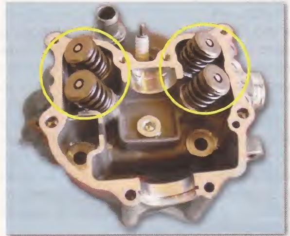
Culata con cuatro válvulas completas
